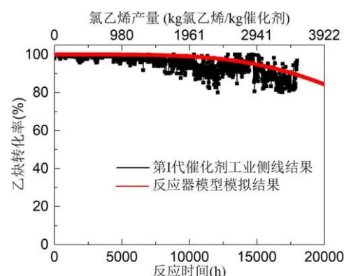
图2 第一代金基催化剂工业侧线
