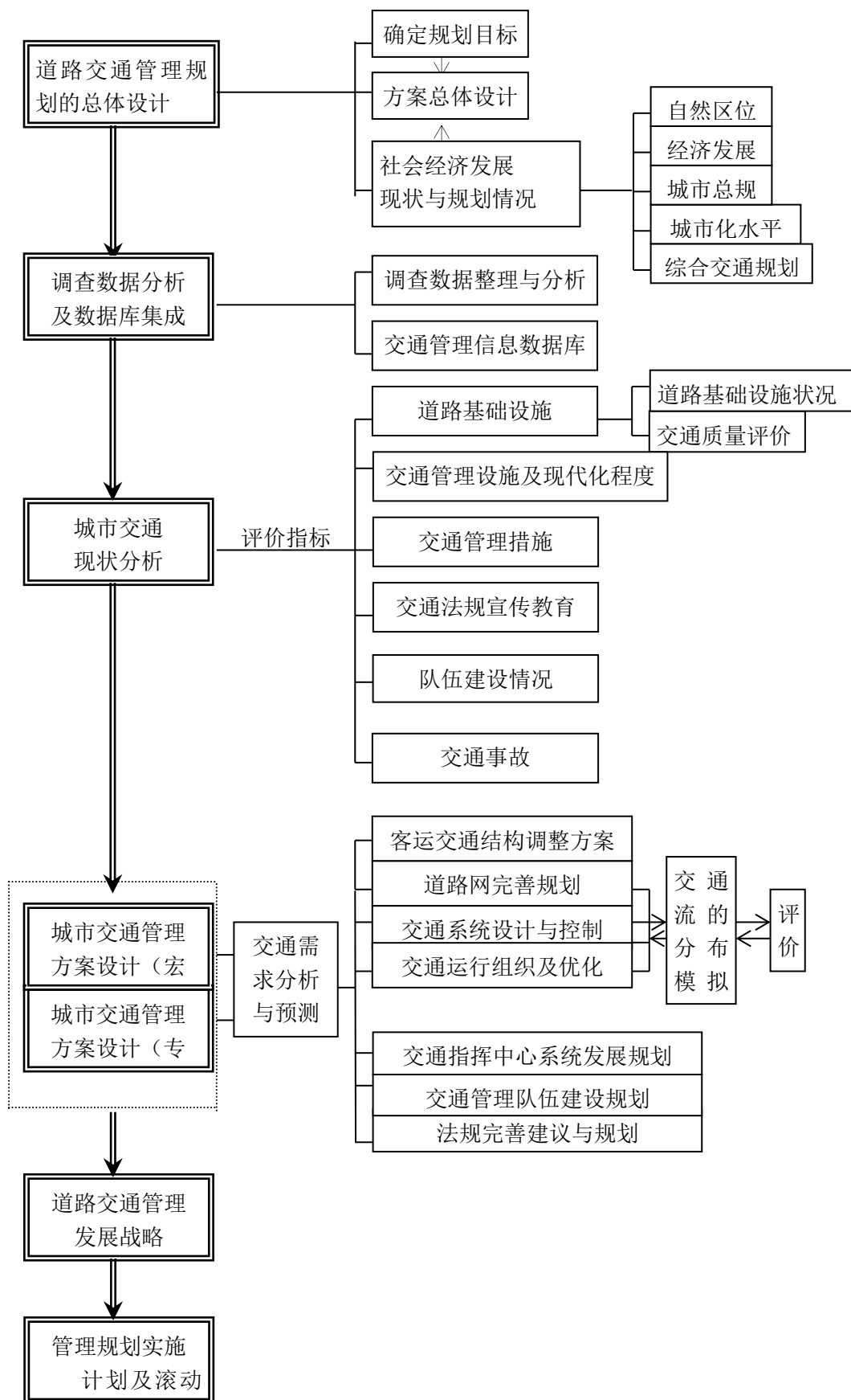
上图 道路交通管理规划技术流程图
