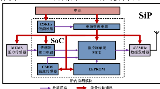
图 1 TPMS 芯片框图(虚线内)
