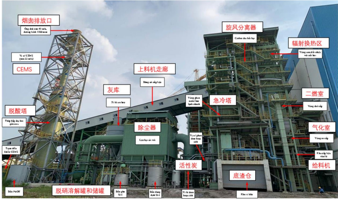
图 2 越南平阳废渣污泥焚烧项目现场图
